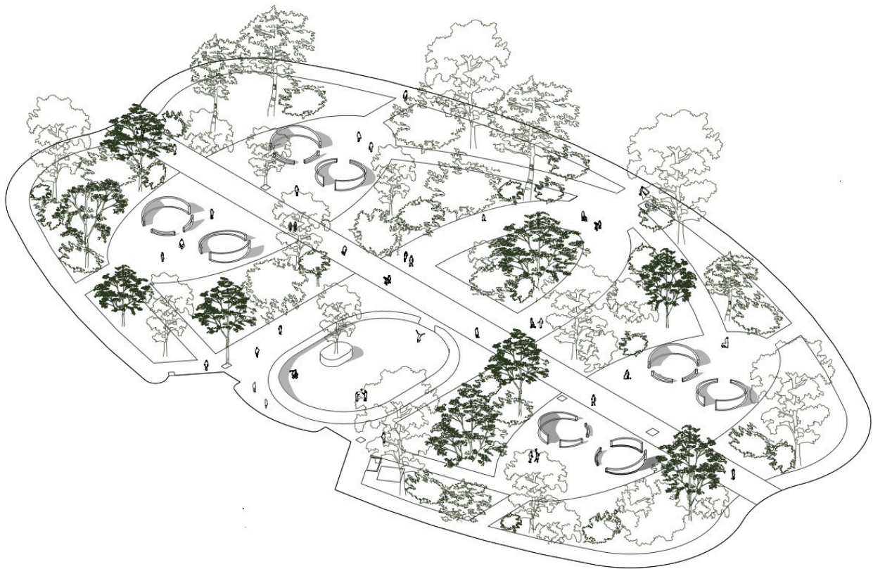
• Imagen 03 - Axonométrico Parque América
