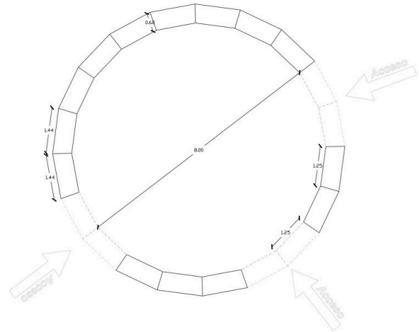
• Imagen 02 - Envolverte en planta
